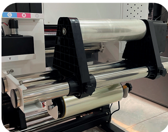
Sistema de desembobinado trasero
